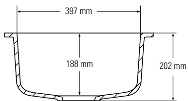
Vista sezione laterale
