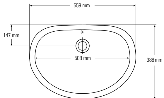
Vista dall'alto * troppopieno
