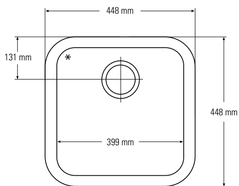
Vista dall'alto * troppopieno
