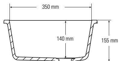
Vista sezione laterale
