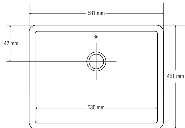
Vista dall'alto * troppopieno
