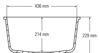
Vista sezione laterale
