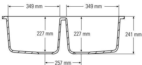
Vista sezione frontale
