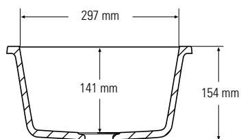
Vista sezione laterale
