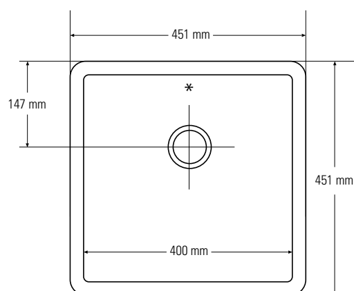
Vista dall'alto * troppopieno
