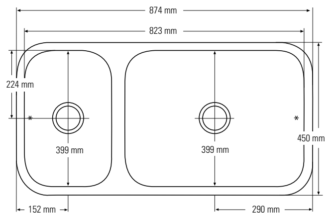
Vista dall'alto * troppopieno
