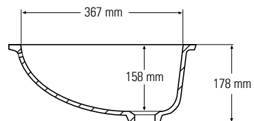
Vista sezione laterale
