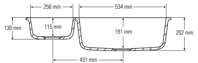
Vista sezione frontale
