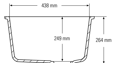
Vista sezione laterale
