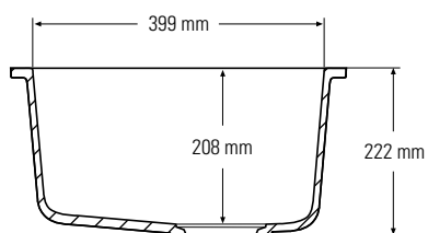
Vista sezione laterale
