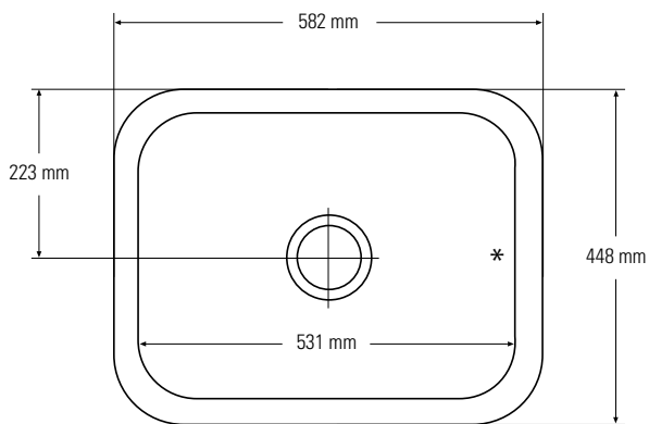
Vista dall'alto * troppopieno
