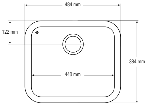
Vista dall'alto * troppopieno
