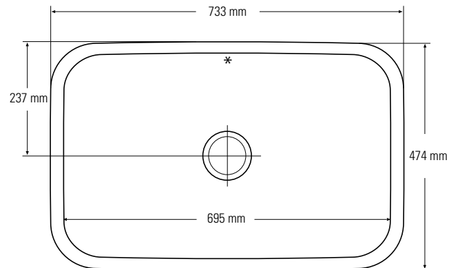
Vista dall'alto * troppopieno
