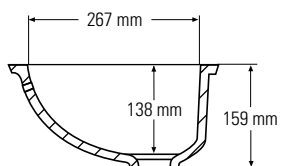
Vista sezione laterale
