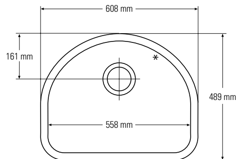
Vista dall'alto * troppopieno
