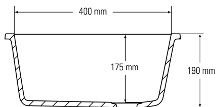
Vista sezione laterale
