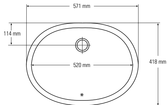
Vista dall'alto * troppopieno
