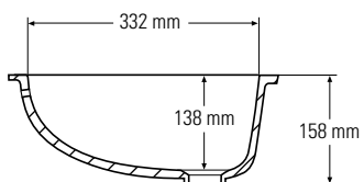
Vista sezione laterale
