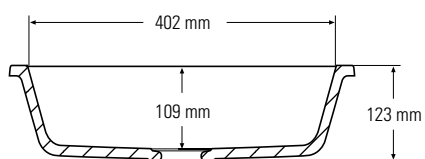
Vista sezione laterale
